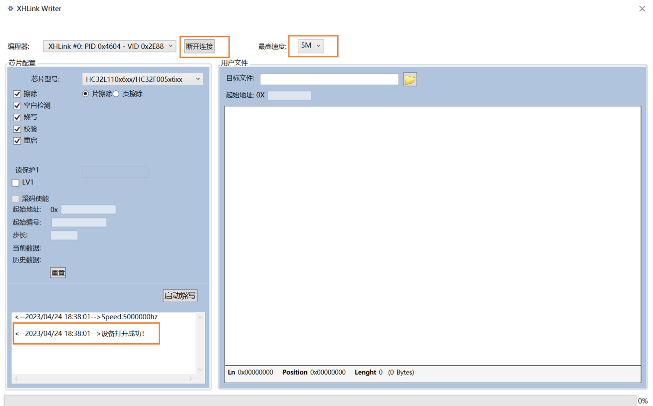
图 4-2 连接成功
